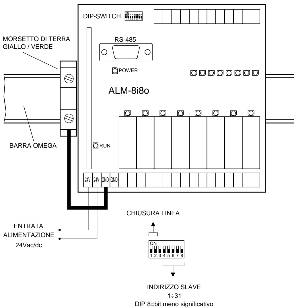
Figura 6. Connessione dell'alimentazione
