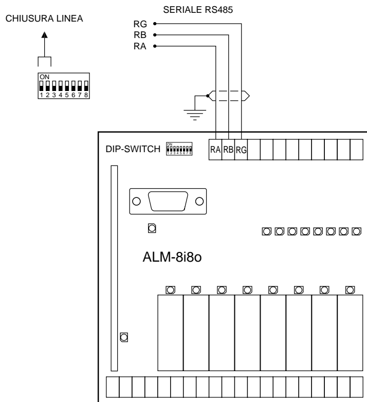
Figura 7. Connessione alla rete RS485
