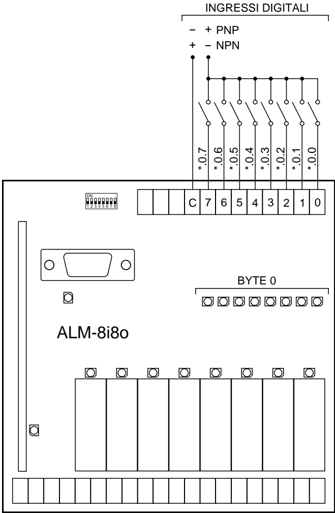
Figura 3. Connessione ingressi digitali
