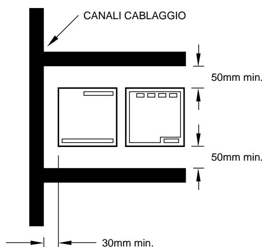
Figura 8. Posizionamento della logica all'interno del quadro
