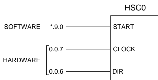
Figura 4. Schema a blocchi HSC0.
