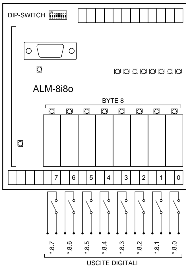
Figura 5. Connessione uscite digitali
