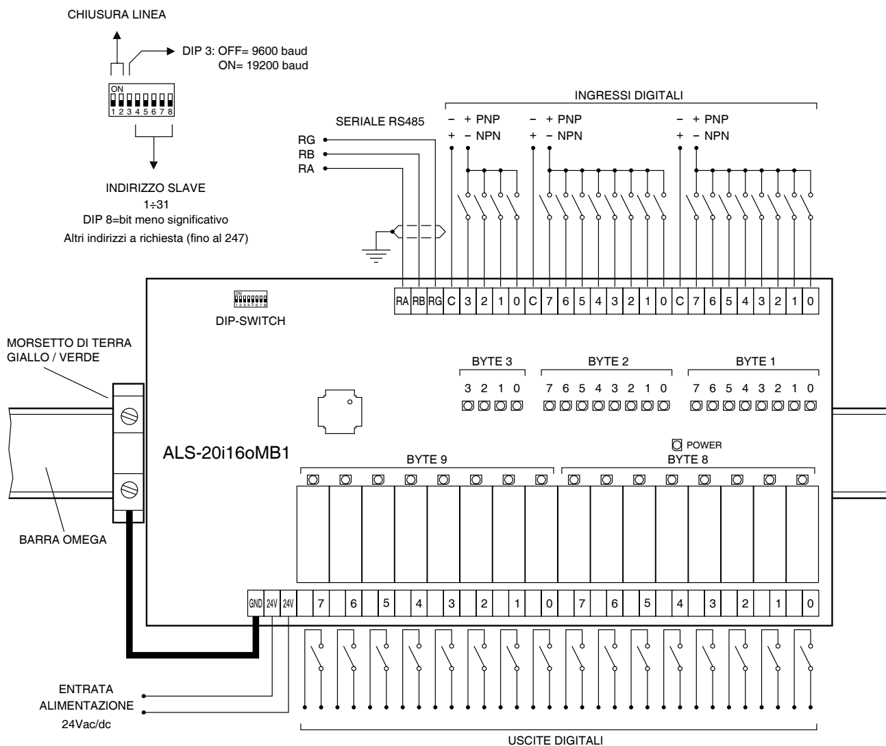
Schema di collegamento ALS-20i16oMB1
