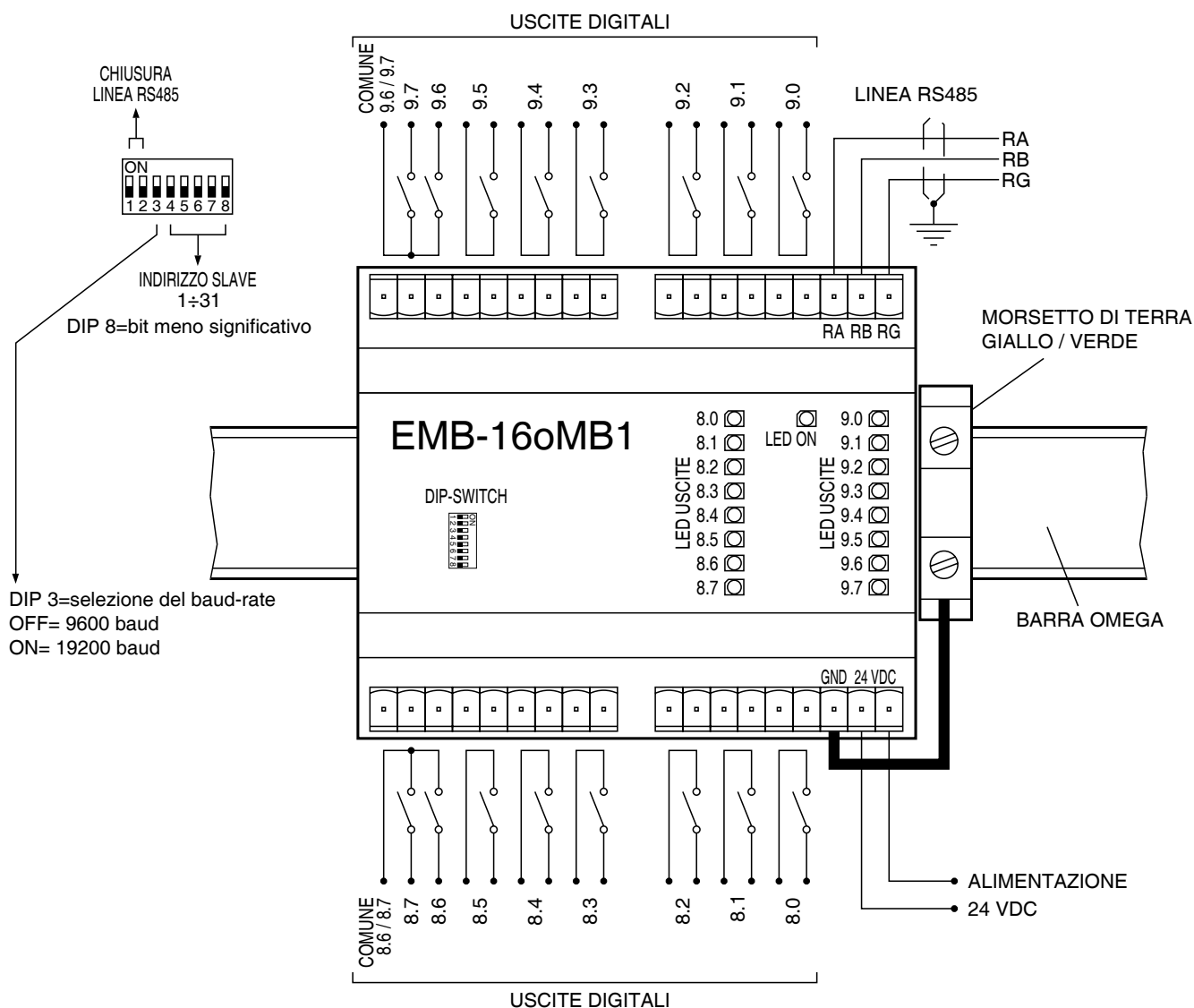
Schema di collegamento EMB-16oMB1
