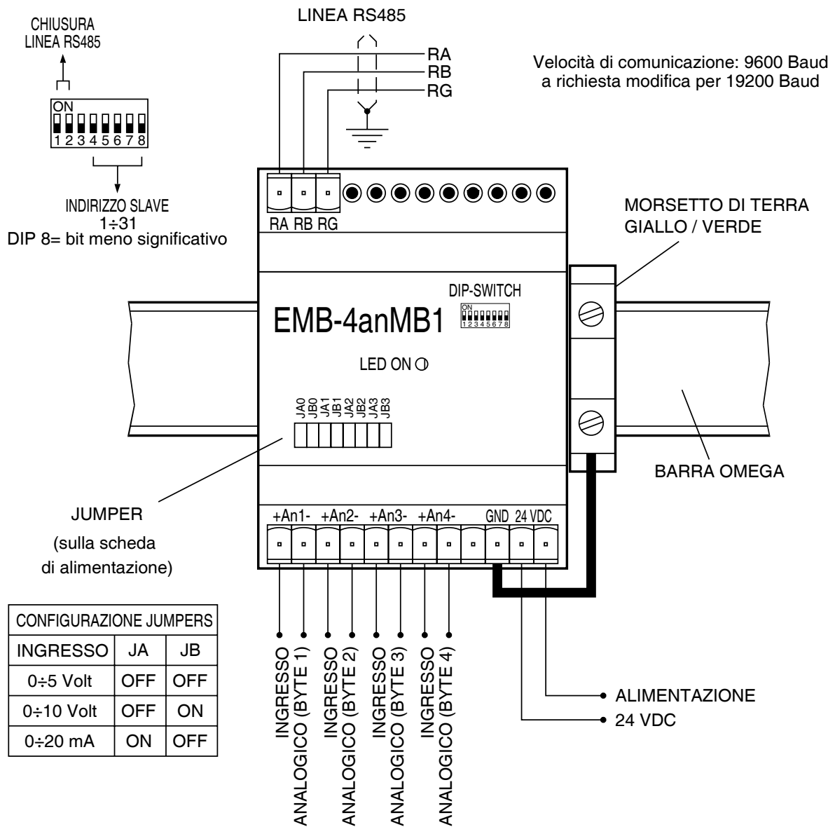
Schema di collegamento EMB-4anMB1
