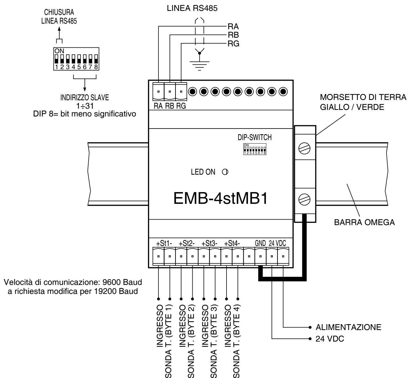
Schema di collegamento EMB-4stMB1
