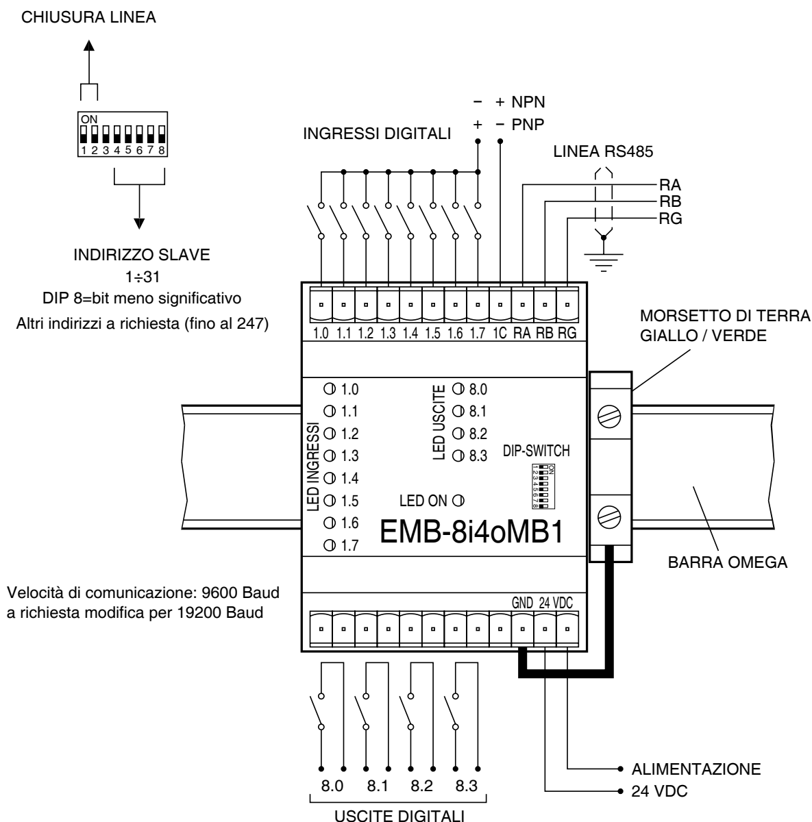
Schema di collegamento EMB-8i4oMB1
