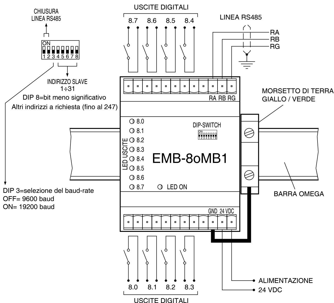
Schema di collegamento EMB-8oMB1
