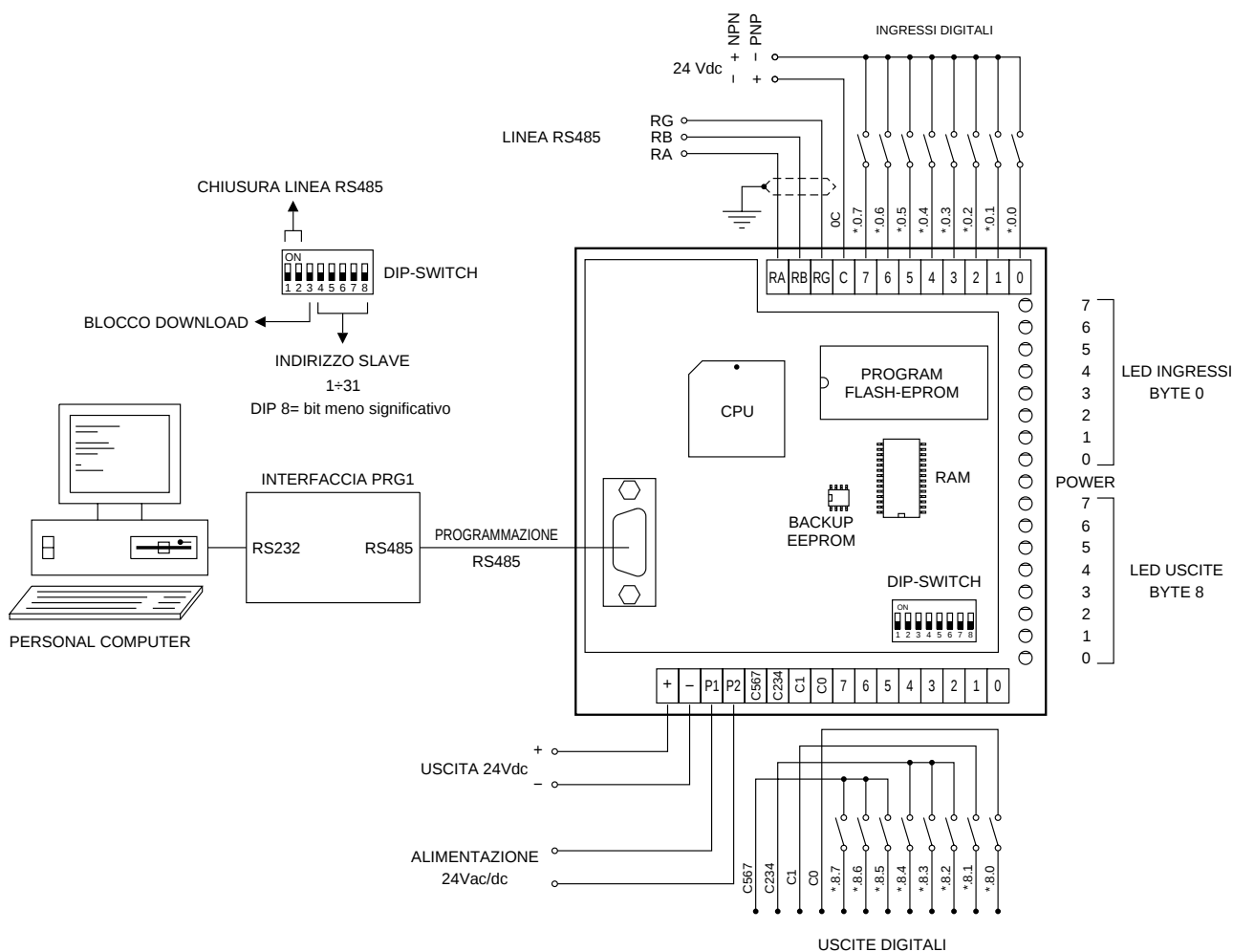
Figura 1. Topologia e cablaggio della ML15LC
