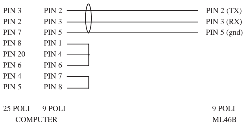
Figura 2. Cavo di connessione ML46B - Computer
