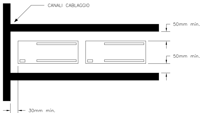
Figura 8. Posizionamento della logica all'interno del quadro
